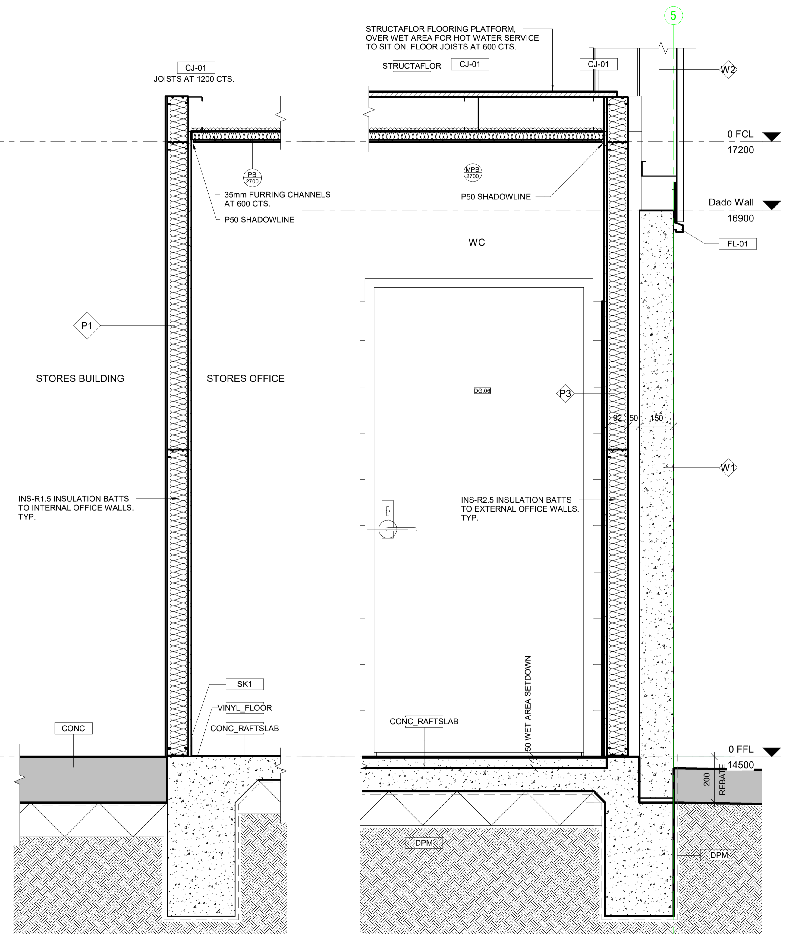
SD.C1 Section Detail SD.C1 1:10
