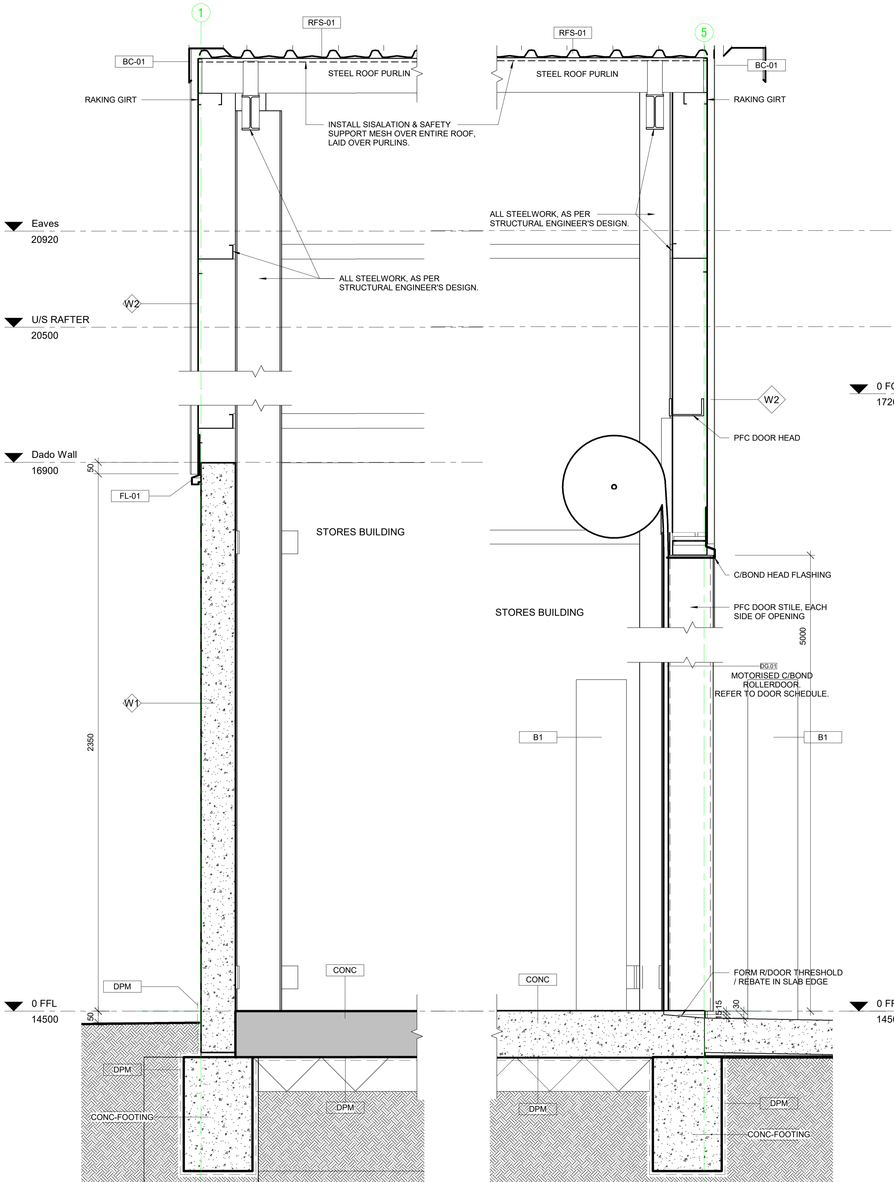
SD.B1 Section Detail SD.B1 1:10
